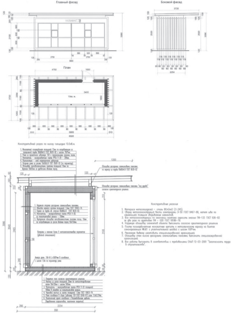
2. Тип 2.3 «Киоск» общая площадь 15 кв. м.
