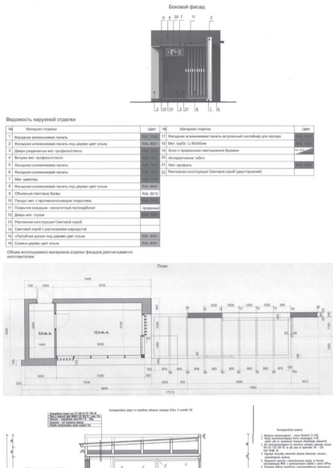
3. Тип 3.3 «Торгово-остановочный комплекс» общая площадь павильона 50 кв. м.
